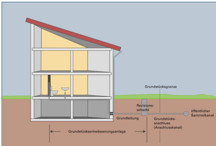
Abb. 1: Im Idealfall werden Abwasserleitungen nicht unterhalb des Gebäudes, sondern entlang der Kellerdecke verlegt. So sind sie von der Prüfpflicht befreit.
